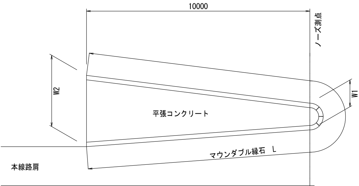
ノーズ標準図 S=1:50
