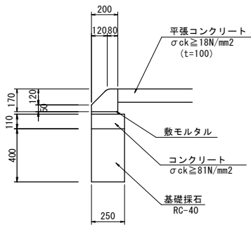
マウンダブル縁石 S=1:20
